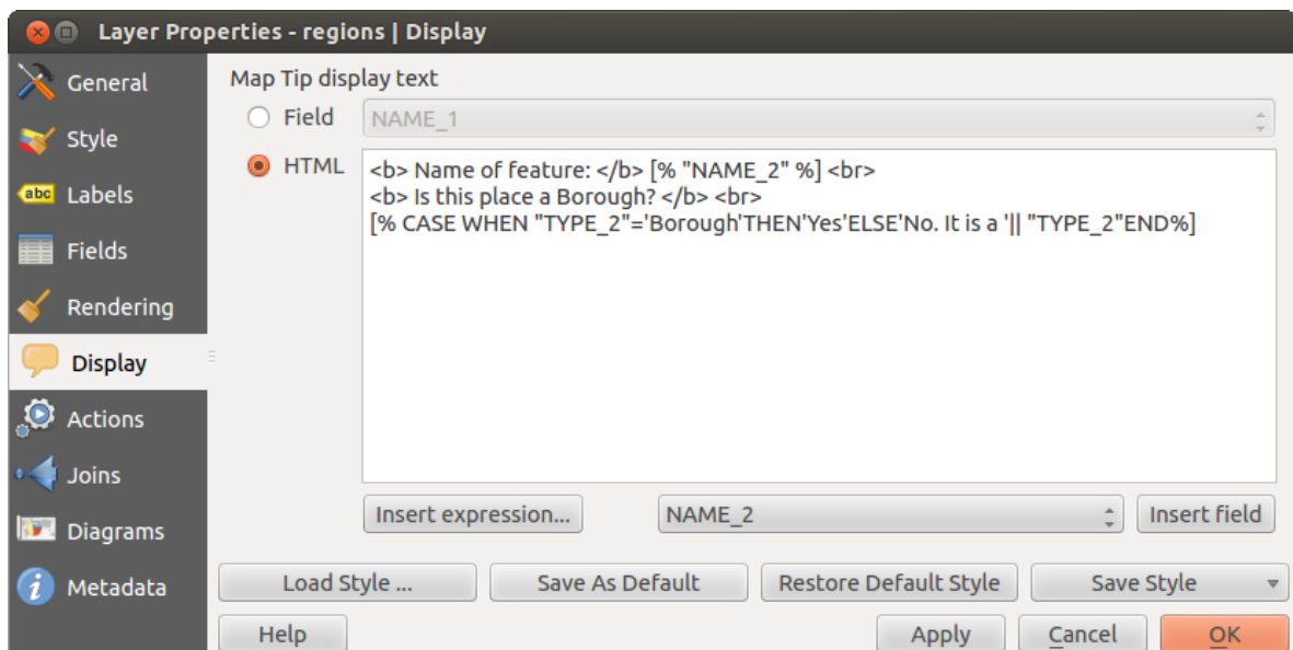
Figure 12.32: Code HTML pour les infobulles 🐧
