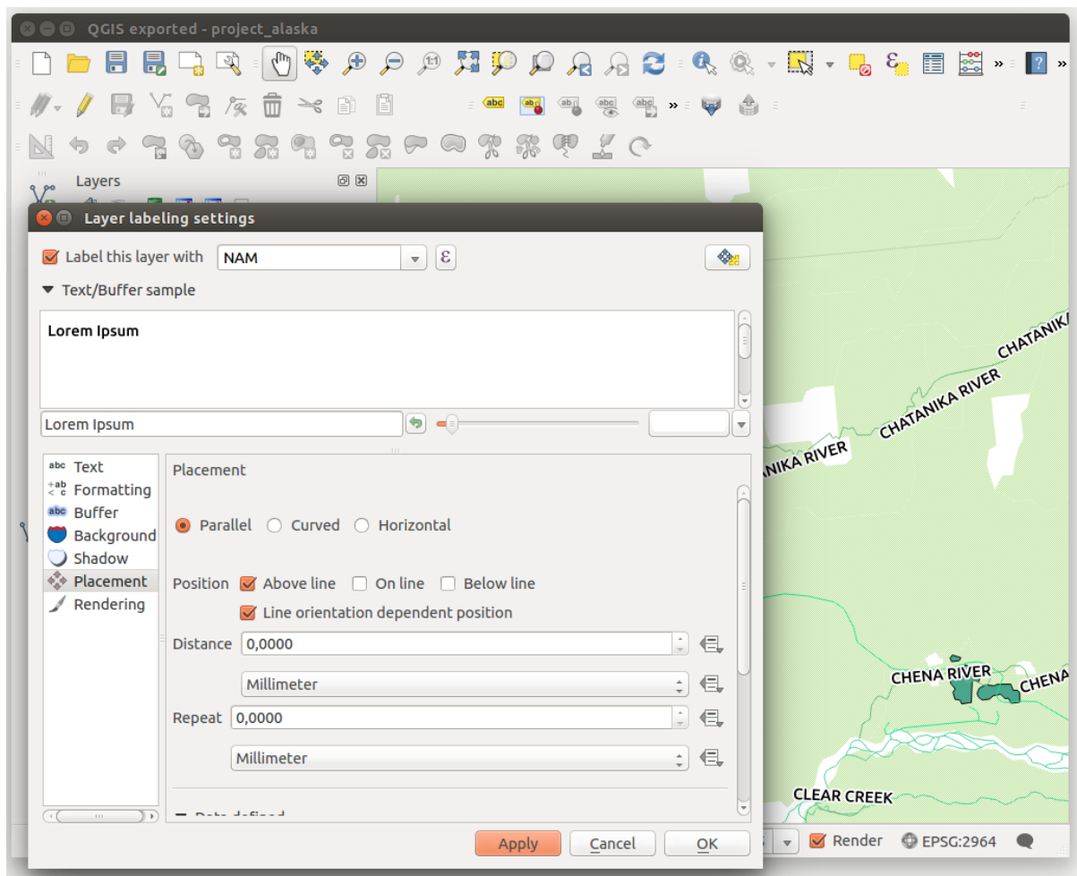
Figure 12.23: Étiquetage d'une couche vectorielle de lignes 🐧
