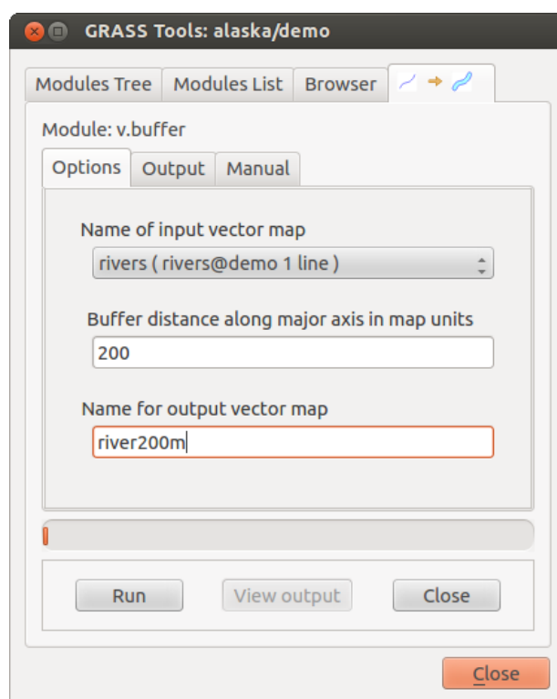
Figure 16.9: Boîte à outils GRASS, onglet Options d'un module 🐧
