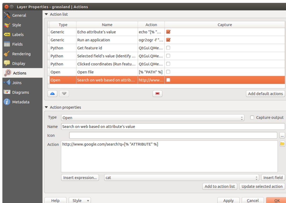
Figure 12.34: Vue d'ensemble de la fenêtre Actions avec quelques exemples d'actions 🐧
