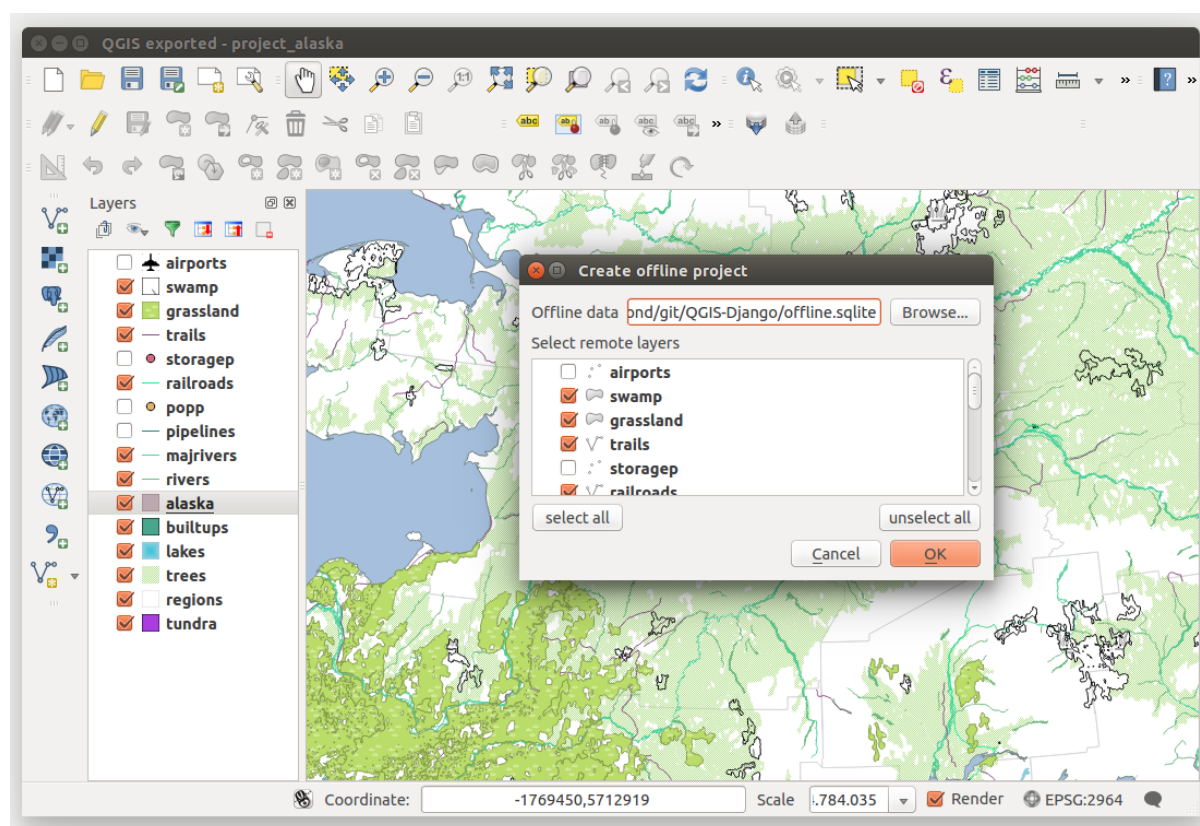
Figure 19.25: Crée un projet hors ligne depuis PostGIS ou des couches WFS
