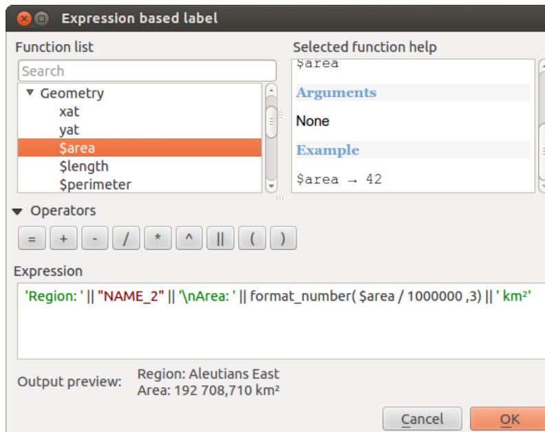
Figure 12.25: Utiliser des expressions pour l'étiquetage 🐧
