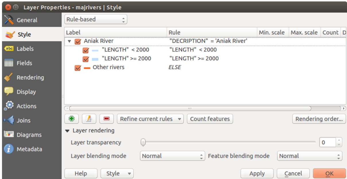
Figure 12.16: Options du mode de rendu par Ensemble de Règles 🐧
