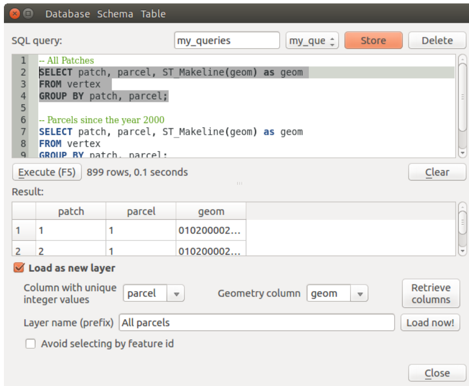
Figure 19.8: Exécution de requêtes dans la fenêtre SQL de DB Manager 🐧
