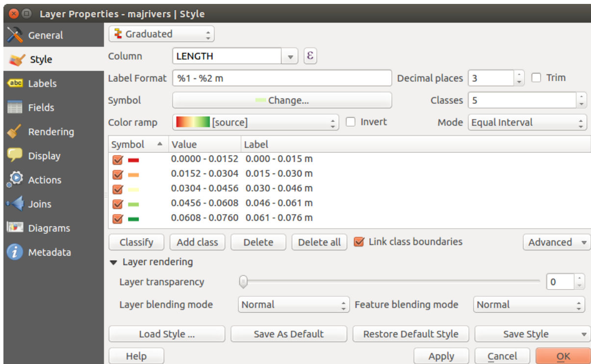
Figure 12.15: Options du mode de rendu Gradué 🐧
