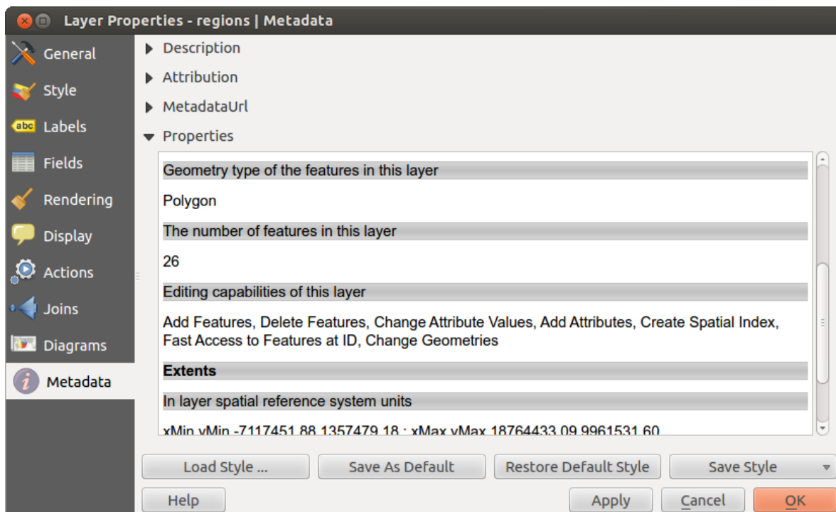
Figure 12.39: Onglet Métadonnées de la fenêtre de Propriétés d'une couche vecteur 🐧
