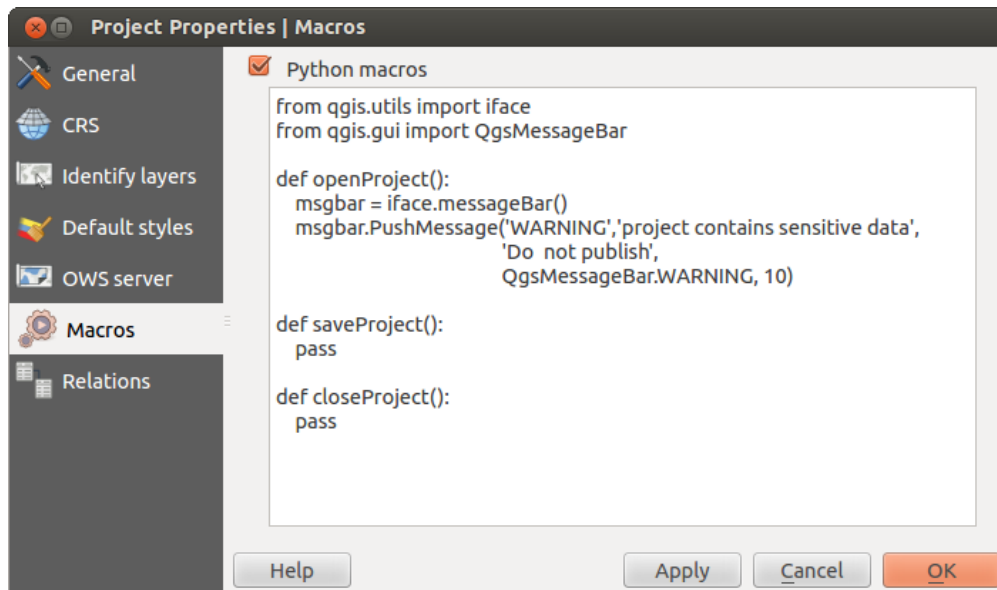
Figure 9.2: Paramètres des macros dans QGIS
